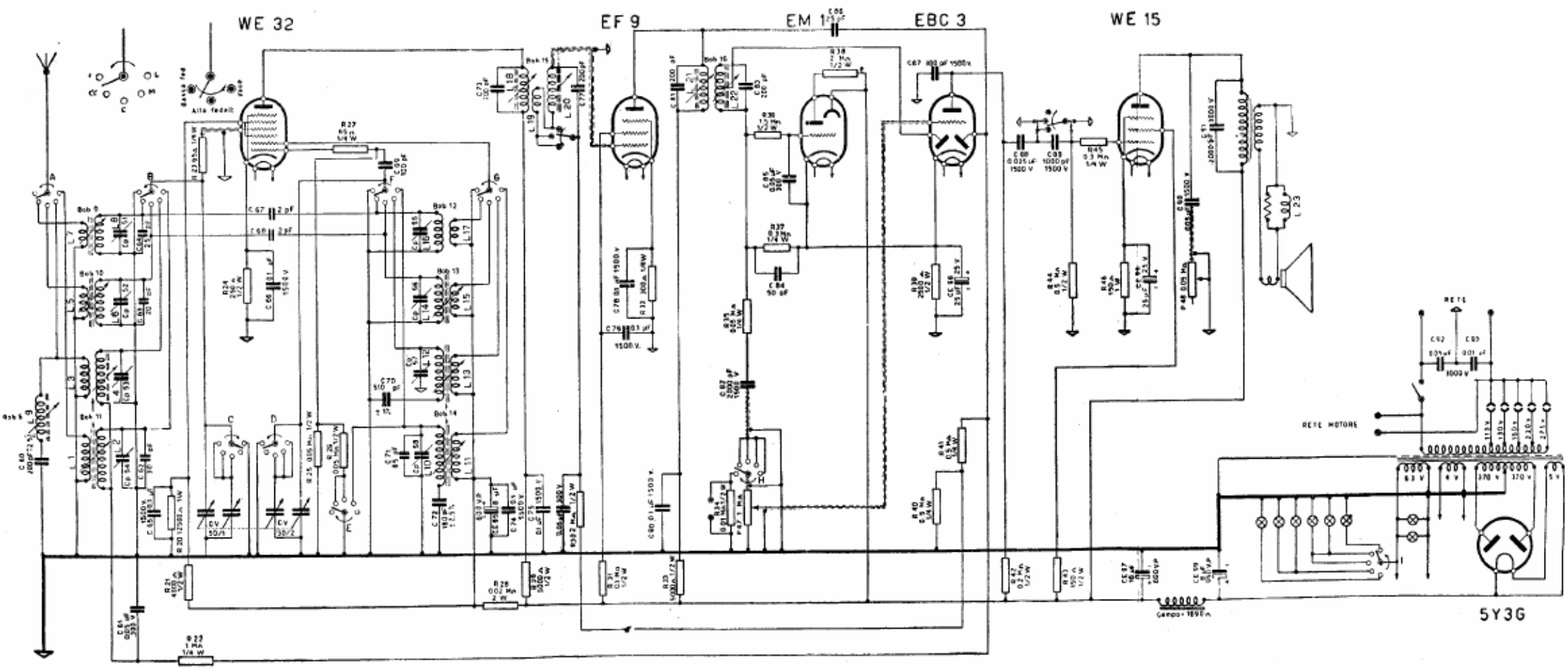
- Moderna supereterodina a 4 gamme d'onda. (Voce del Padrone, telaio mod. 531).
